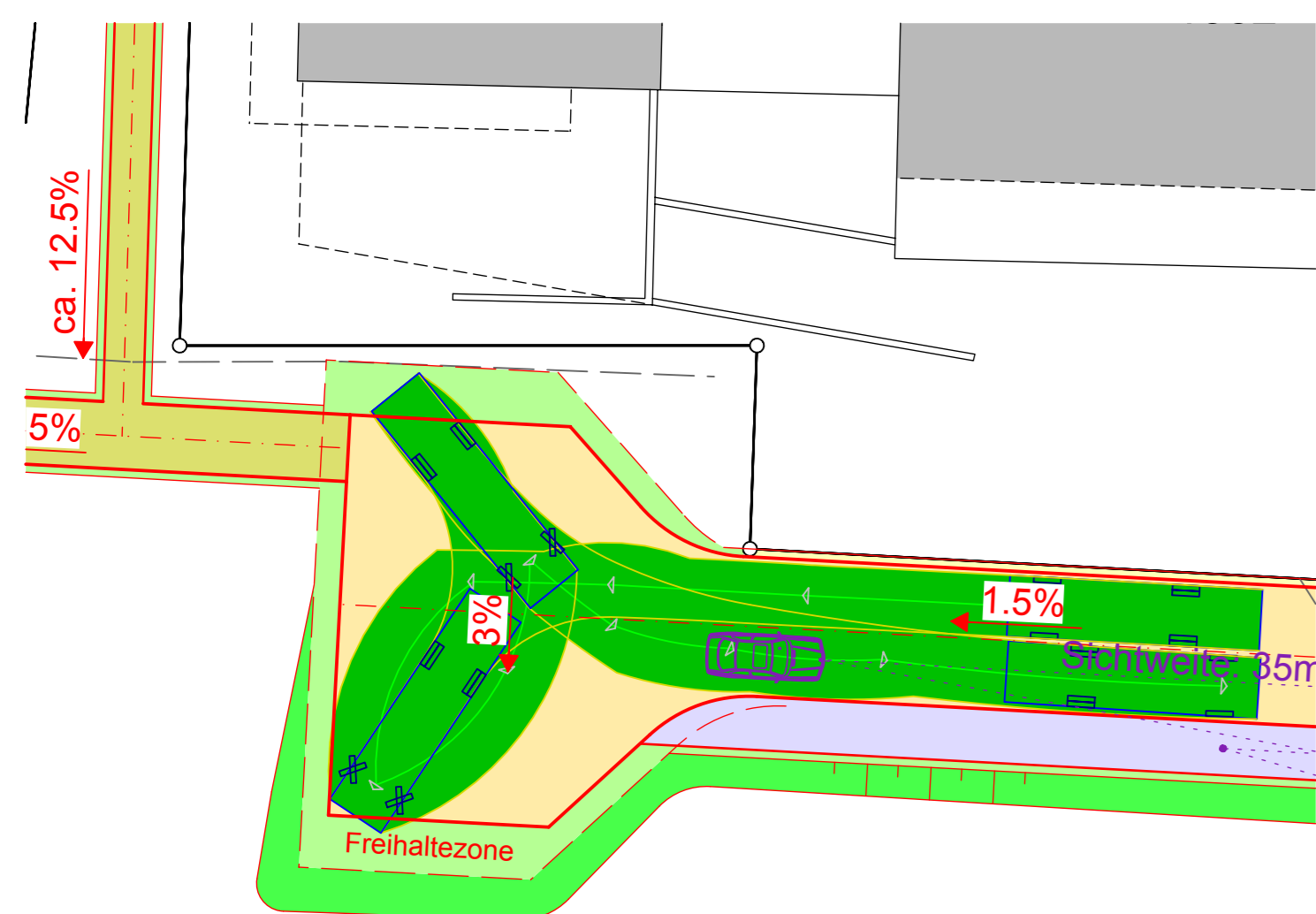
Situation 1 : 250, Wendemanöver (kleiner LKW, V=10km/h)
